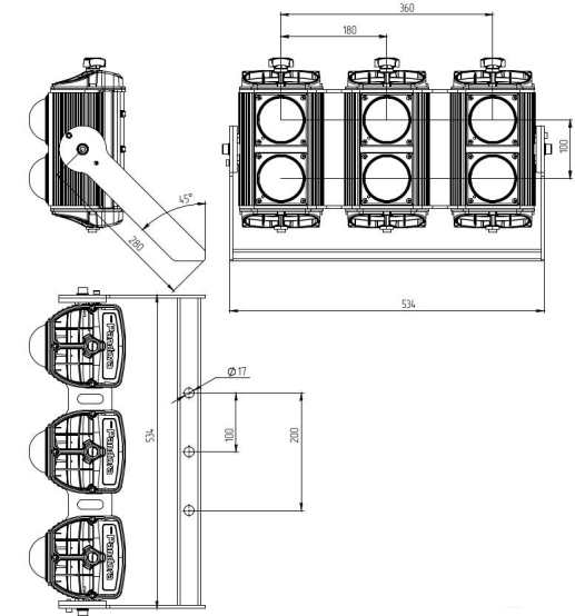
Рисунок 2. Габаритный чертеж
